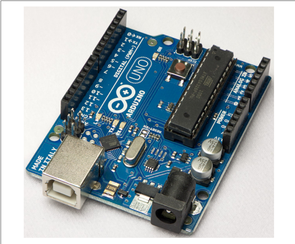
Figure 4-7. Arduino Uno controller
